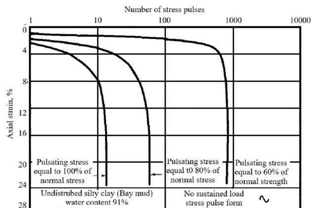
Рисунок 8. Деформации грунта под воздействием вибрационной нагрузки в направлении одной оси [19]
