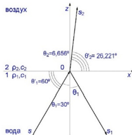
Рис. 4. Схема падения звуковой волны на границу двух сред: воды и воздуха.
