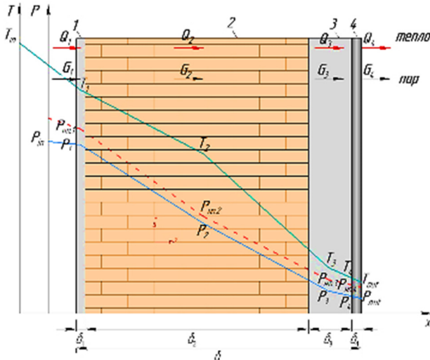
Рисунок 1 – Расчетная схема ограждающей конструкции
