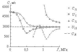
Рис. 1. Дисперсионные характеристики стержня для симметричных колебаний.
