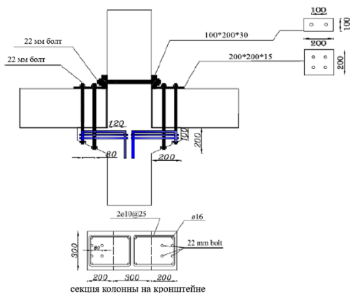
Рис. 4 Соединение на болтах
