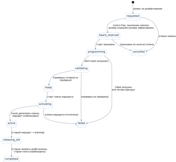
Рисунок 2 — Машина состояний попытки развертывания с условиями переходов
