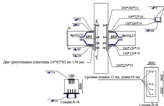
Рис. 3 Соединение без швеллера и сварки
