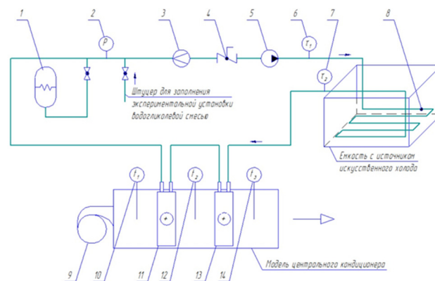
1 – гидроаккумулятор; 2 – манометр; 3 – преобразователь расхода электромагнитный; 4 – клапан балансировочный ручной; 5 – насос циркуляционный; 6, 7, 10, 12, 14 – термпреобразователи сопротивления; 8 – теплообменник источника естественного холода; 9 – вентилятор модели центрального кондиционера; 11, 13 – водо-воздушные теплообменники блока воздухоохладителя 1-й и 2-й ступеней модели Рис. 1 – Принципиальная схема установки [2]
