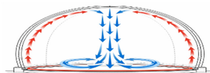
Рис. 2. Аэродинамическая схема торoidalного свободно-конвективного течения в объеме РПУ
