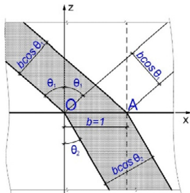
Рис. 1. Принцип прохождения звукового луча, имеющего поперечное сечение, через границу двух сред в методе сосредоточенных параметров
