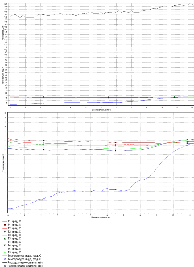
Рис. 5 – Графики изменения температуры воздуха, хладоносителя, льда и расхода хладоносителя от времени (S=0,09 м 2 )
