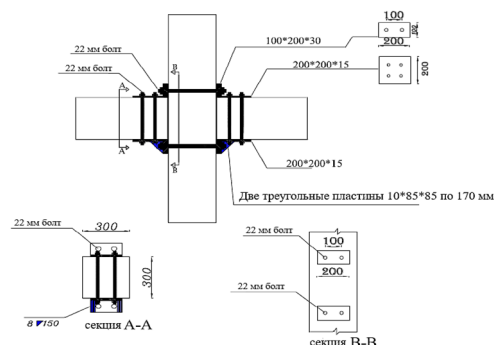
Рис. 2 Болтовое соединение без каркаса
