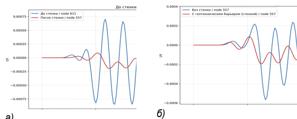
Рисунок 8 а) Сравнение амплитуд вертикальных перемещений грунта «до стенки» и «за стенкой»; б) Сравнение амплитуд вертикальных перемещений грунта без наличия стенки (без геотехнического барьера) – синий график; со стенкой (геотехническим барьером) – красный график. Точка за стенкой.
