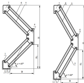
Рисунок 3 – Параметры коленчатого подъёмника при углах \alpha = 45^\circ и \alpha = 60^\circ . (обозначения те же, что и на рис. 2)
