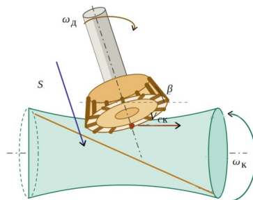
Рисунок 1 — Относительное движение зуборезного долбяка и гиперboloидной заготовки при зуботочении
