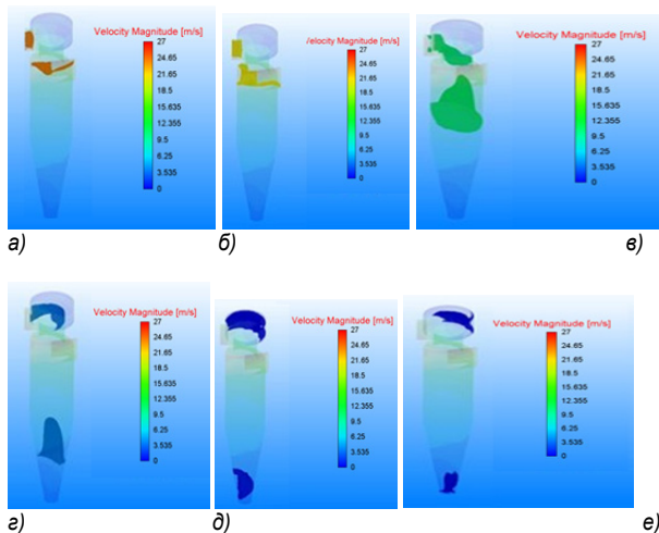
Рис. 5. Зоны определенных значений скоростей: а) 22 м/с; б) 20 м/с; в) 15 м/с; г) 7 м/с; д) 5 м/с; е) 3 м/с
