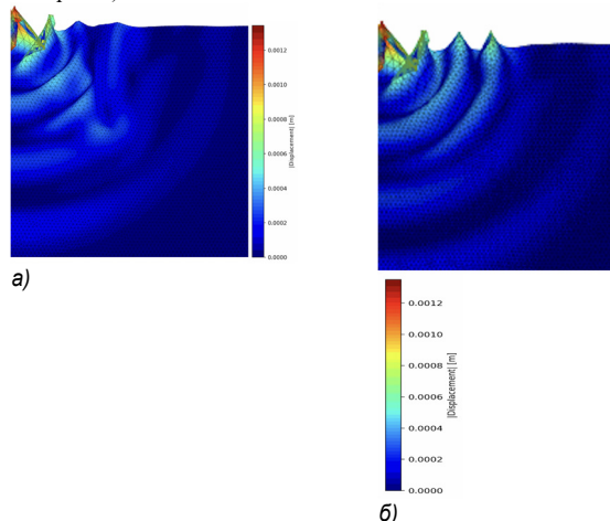
Рисунок 7 Сопоставление амплитуд и деформированных схем на участке между источником динамического воздействия и стенкой: а) есть разделительная стенка; б) стенка отсутствует.
