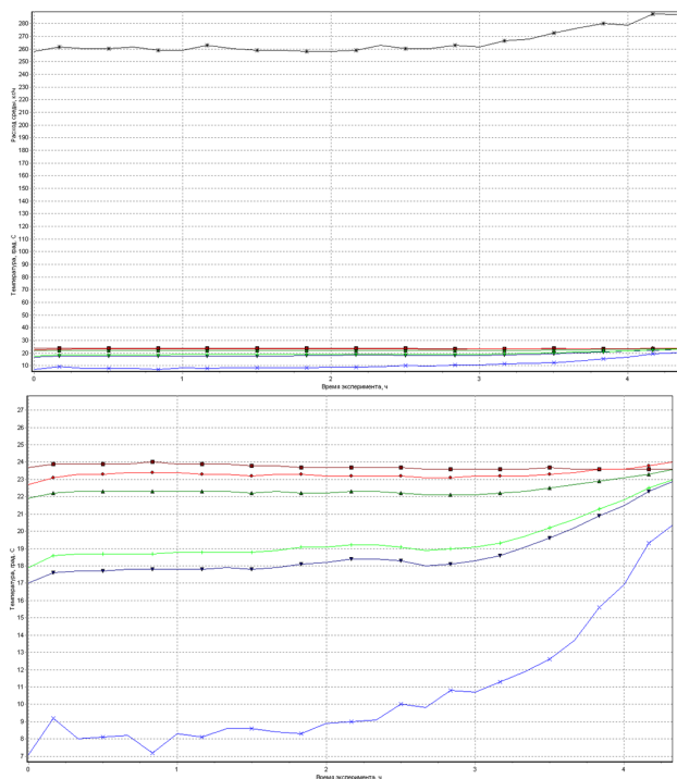
Рис. 6 – Графики изменения температуры воздуха, хладоносителя, льда и расхода хладоносителя от времени ( S=0,181 \text{ м}^2 )
