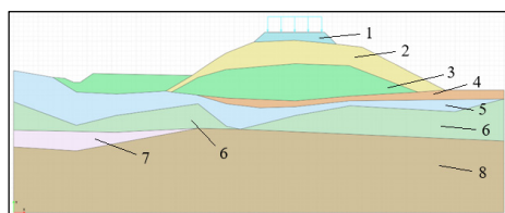
Рисунок 3 – Графическая схема поперечного профиля с мерзлым грунтом 1 – щебень; 2 – песок гравелистый; 3 – щебенистый грунт; 4 – торф; 5 – супесь; 6 – супесь мерзлая; 7 – супесь гравелистая мерзлая; 8 – песок гравелистый мерзлый Источник: составлено автором
