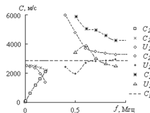
Рис. 2. Дисперсионные характеристики стержня для изгибных колебаний.
