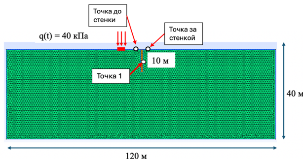
Рисунок 3 Тестовая расчетная схема с указанием точек для контроля колебаний.
