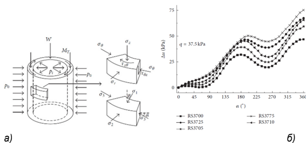
а) Испытание на крутильный сдвиг с возможностью вращения всех осей а) напряженно-деформированное состояние образца [11], б) развитие порового давления по мере возрастания угла \alpha между главными напряжениями и вертикальной осью [11]
