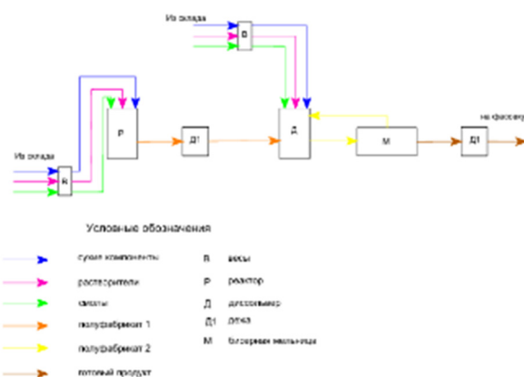
Рис.1. Принципиальная технологическая схема производства ЛКМ
