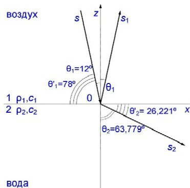
Рис. 3. Схема падения звуковой волны на границу двух сред: воздуха и воды.
