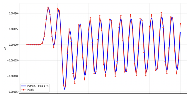
Рисунок 4 Сопоставление перемещений узла по оси X, м.
