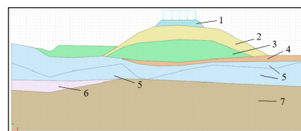
Рисунок 5 – Графическая схема поперечного профиля с талым грунтом 1 – щебень; 2 – песок гравелистый; 3 – щебенистый грунт; 4 – торф; 5 – супесь; 6 – супесь гравелистая мерзлая; 7 – песок гравелистый мерзлый Источник: составлено автором
