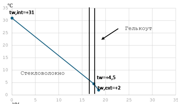
Рис.1. Распределение температур по толщине оболочки купола при внешнем охлаждении
