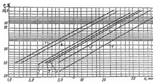
Рис. 7. Фракционная эффективность очистки циклонов [6]: 1 – СК-ЦН-34; 2 – ЦН-11; 3 – ЦН-15; 4 – ЦН-15у; 5 – ЦН-24; 6 – СДК-ЦН-33; 7 – СДК-ЦН-33-400
