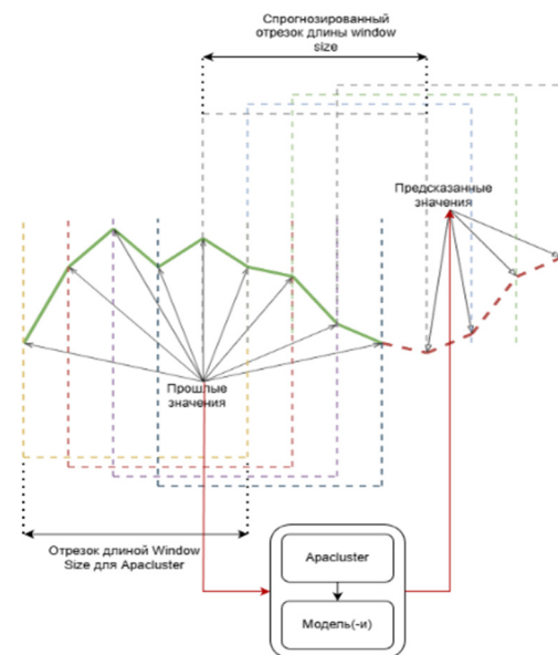
Рисунок 3. Результат прогноза AраLMS (источник: составлено авторами)
