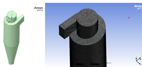
а) б) Рис.3. Геометрическая модель (а) и модель с расчетной сеткой (б) циклона
