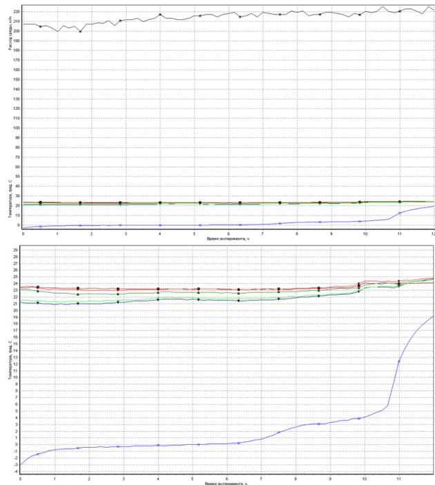
Рис. 7 – Графики изменения температуры воздуха, хладоносителя, льда и расхода хладоносителя от времени ( S=0,045 \text{ м}^2 )
