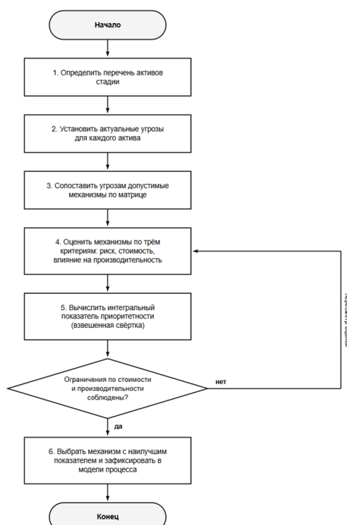
Рисунок 2 – Блок-схема алгоритма отбора защитного механизма
