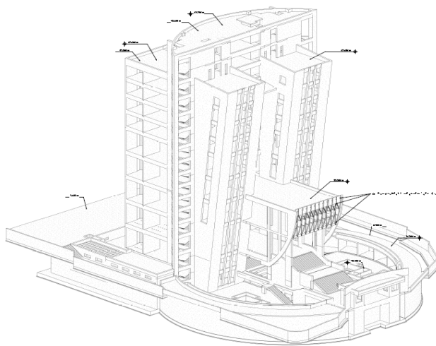
Рис.4. Каркас здания
