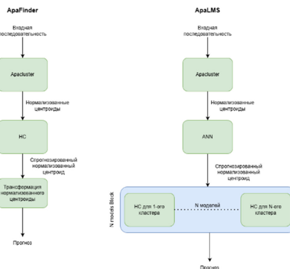
Рисунок 1. Сравнение схем AraFinder и AraLMS (источник: составлено авторами)
