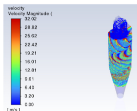
Рис. 6. Распределение скорости в циклоне
