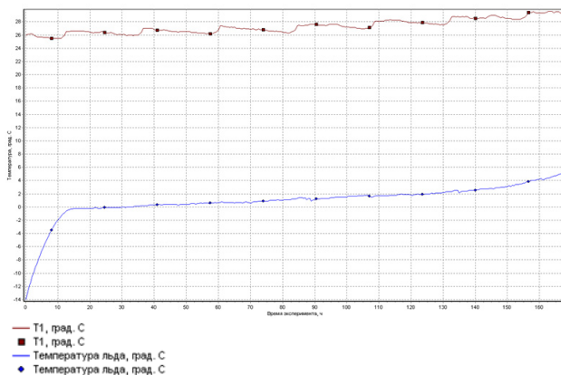
Рис. 8 – Графическая зависимость изменения температуры воздуха в помещении и льда (талой воды) во времени
