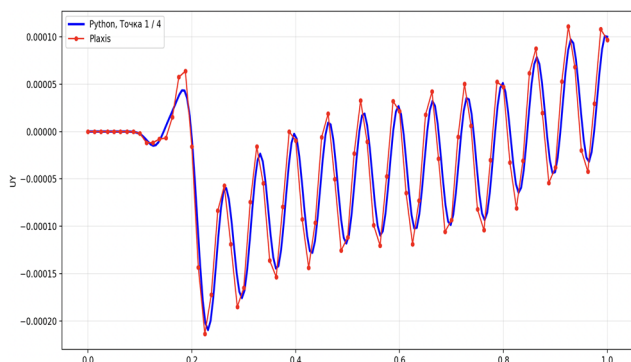
Рисунок 5 Сопоставление перемещений узла по оси Y, м
