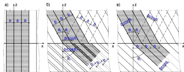
Рис. 2. Схемы падения звуковых лучей на границу двух сред: а – падение под углом в 90^\circ ; б – нарушение условия неразрывности из-за наложения звуковых лучей, сохраняющих свою ширину при изменении угла их распространения (выделено тёмно-серым цветом); в – косое падение звуковых лучей на границу сред, условие неразрывности соблюдается
