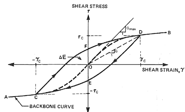
Рисунок 6. Кривая, описывающая напряженно-деформированное состояние грунта за первый цикл колебаний [20]
