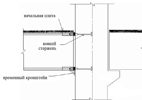
Рис. 1 Вязкие соединители
