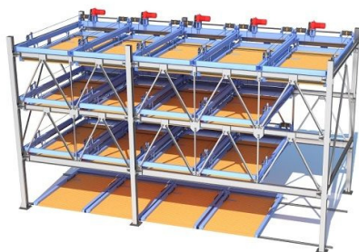
Рис. 5 Пазловая парковка
