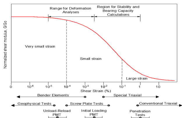
Рисунок 4. Кривая снижения жесткости в диапазонах деформаций с указанием методов испытаний [18]
