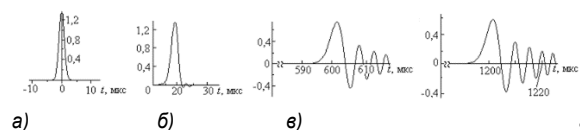
Рис. 4. Дисперсионные искажения формы УЗ импульса: а – x = 0 м, б – x = 0,1 м, в – x = 3 м, г – x = 6 м,
