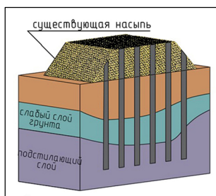
Рисунок 7 – Усиление существующей насыпи с использованием щебеночных свай Источник: [19]
