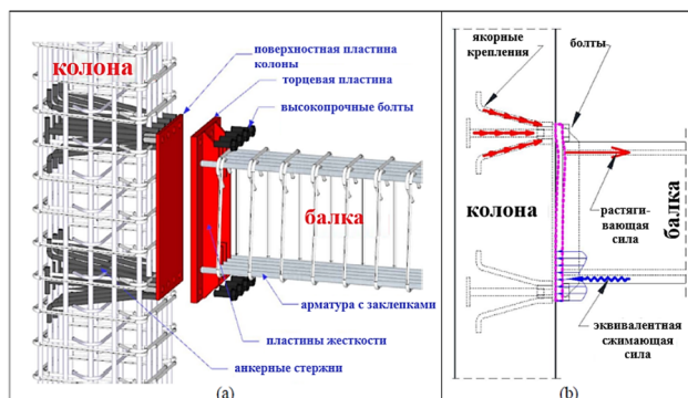
Рис. 5 Общая схема сборного соединения: (a) геометрия соединения балки с колонной; (b) общий механизм передачи нагрузки
