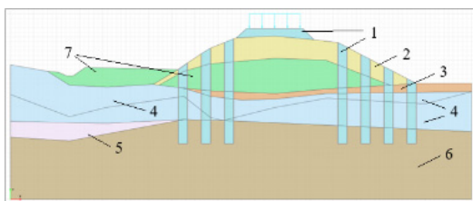
Рисунок 8 - Поперечного профиля насыпи со усилением щебеночными сваями 1 — щебень; 2 — песок гравелистый; 3 — торф; 4 — супесь; 5 — супесь гравелистая мерзлая; 6 — песок гравелистый мерзлый; 7 — щебенчатый грунт Источник: составлено автором
