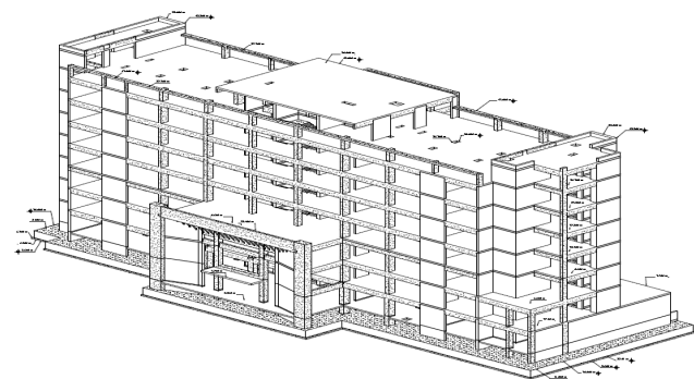
Рис.2. Каркас здания
