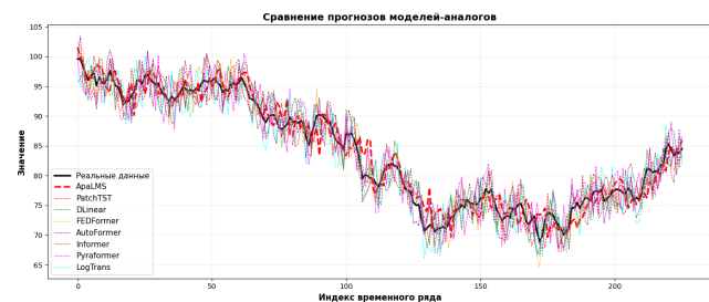
Рисунок 4. Сопоставление реальных данных, и прогнозов моделей аналогов и AраLMS для ALRS (источник: составлено авторами)
