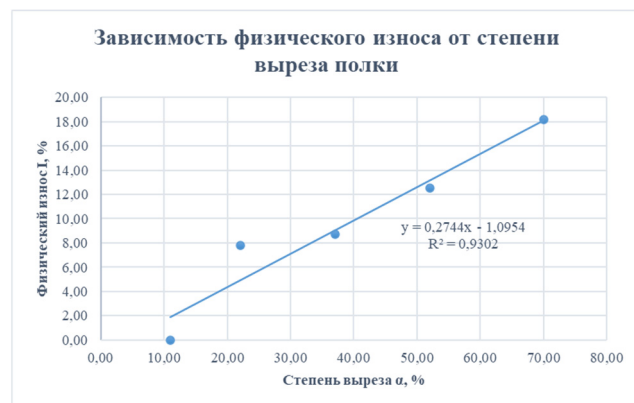
Рисунок 3. Зависимость физического износа от степени выреза полки I = f(\alpha)
