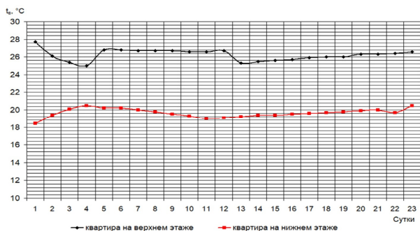
Рисунок 2. Среднесуточные значения температуры воздуха в квартирах
