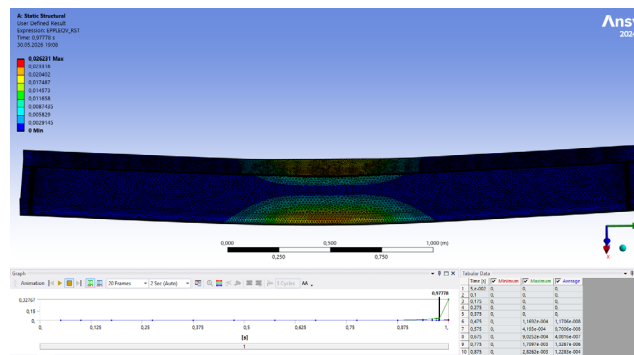
Рисунок 1. Эталонная балка: поле эквивалентной пластической деформации EPPLEQV в предельном состоянии
