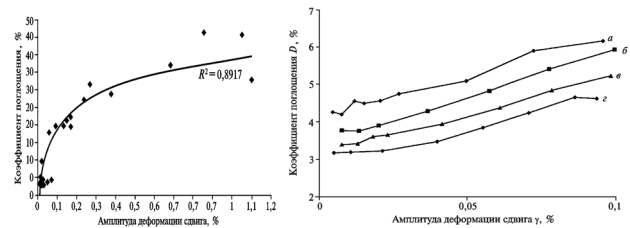
А) Рисунок 5. А) Изменение поглощения глинистых грунтов в диапазоне средних деформаций сдвига по данным испытаний на резонансной колонке и динамического крутильного сдвига [5]. Б) Постепенное снижение коэффициента поглощения суглинка с увеличением продолжительности консолидации: а – 7200 с; б – 14 400 с; в – 28 800 с; г – 56 400 с [5]
