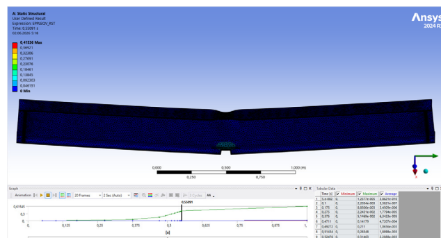
Рисунок 2. Поле эквивалентной пластической деформации EPPLEQV для балки с вырезом полки (точка B3)
