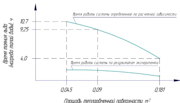
Рисунок 9 – Результаты сравнения времени работы системы кондиционирования, определенного по расчетной зависимости и по результатам эксперимента
