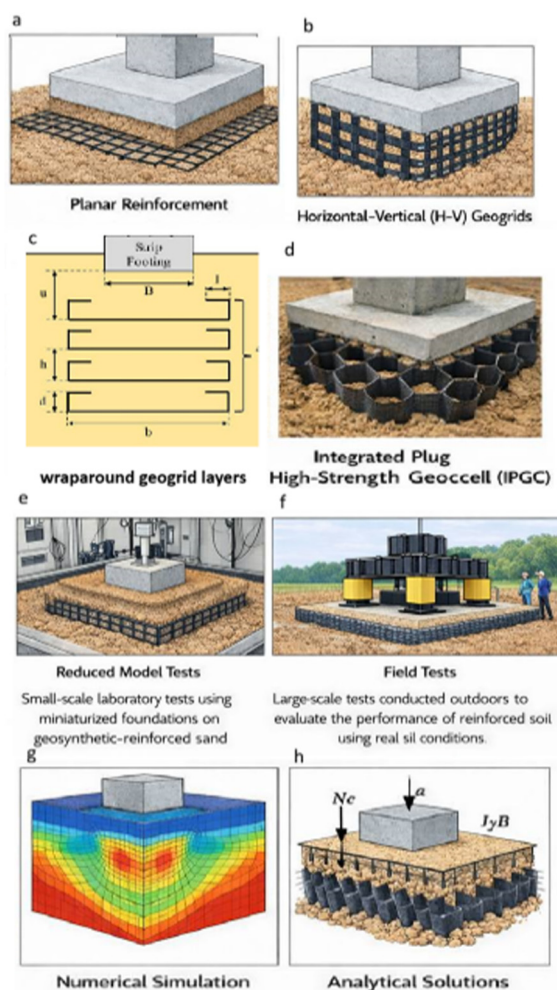
Рис. 1. Методы армирования оснований и подходы к их исследованию
