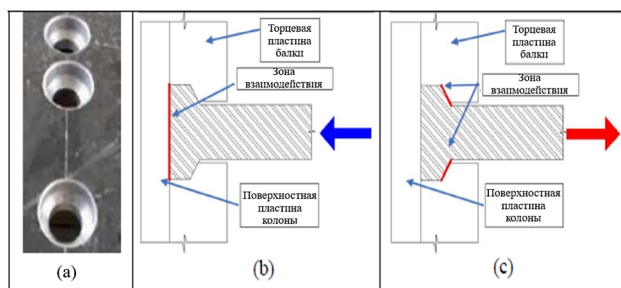
Рис. 6 Детали арматуры: (a) отверстие для арматуры с головкой заклепки; (b) механизм передачи нагрузки при сжатии (c) механизм передачи нагрузки при растяжении
