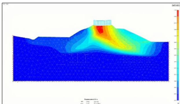
Рисунок 6 – Результат расчета поперечного профиля насыпи на оттаявших грунтах Источник: составлено автором
