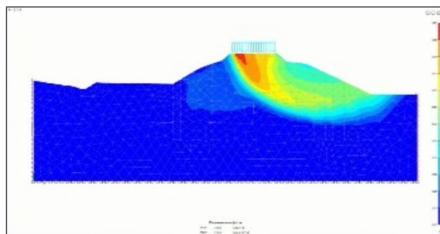
Рисунок 9 – Результат расчета поперечного профиля насыпи на оттаявших грунтах с сооружением щебеночных свай Источник: составлено автором
