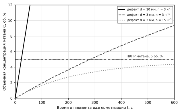
Рис. 2. Нарастание объемной концентрации метана в помещении объемом 30 м 3
