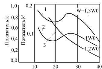
Рисунок 3. Влияние содержания в грунтах глинистых частиц на их тиксотропное разупрочнение: 1, 2 – при вибрировании с частотой f = 50 \text{ Гц} , 3 – при одиночном ударе [6]
