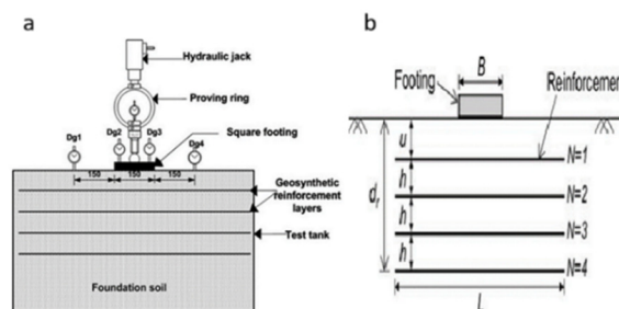
Рис. 3. Схемы испытаний и расчетной модели армированного основания: (а) схема лабораторной установки для испытаний модели фундамента на армированном основании; (б) расчетная схема армированного основания с послойным расположением армирующих элементов.
