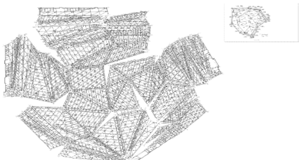
Рис.3 Оперный театр в Гуанчжоу, развернутый макет основной стальной конструкции.
