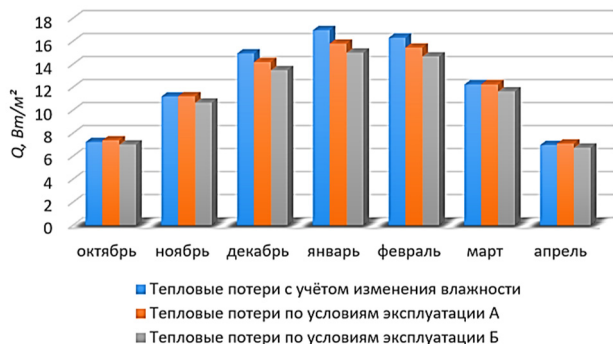
Рисунок 2 – Тепловые потери для ограждающей конструкции панельного здания с утеплителем ТЕХНОФАС ПРОФ
