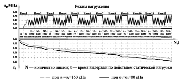
Рисунок 7. Развитие вертикальной деформации в зависимости от режима нагружения [10]
