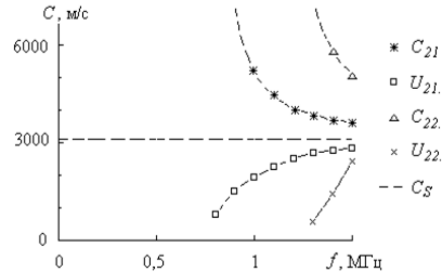
Рис. 3. Дисперсионные характеристики стержней для крутильных колебаний
