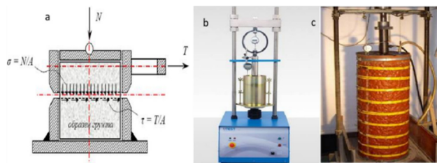
Рис. 2. распространенные методы тестирования образцов армированного грунта.
