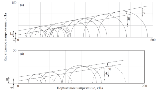
Рисунок 2. Диаграмма Кулона–Мора по результатам статических (сплошная линия) и динамических (пунктирная линия) трехосных испытаний для образцов модельной глины легкой пылеватой тугопластичной (А) и глины тяжелой текучепластичной (Б) [4]
