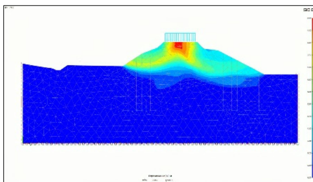
Рисунок 4 – Результат расчета поперечного профиля насыпи Дальневосточной железной дороги, расположенной на мерзлых грунтах Источник: составлено автором
