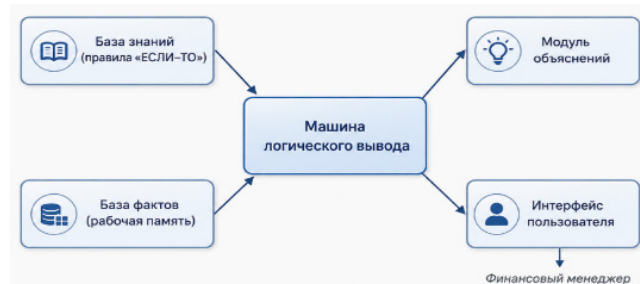
Рис. 1. Обобщенная архитектура экспертной системы
